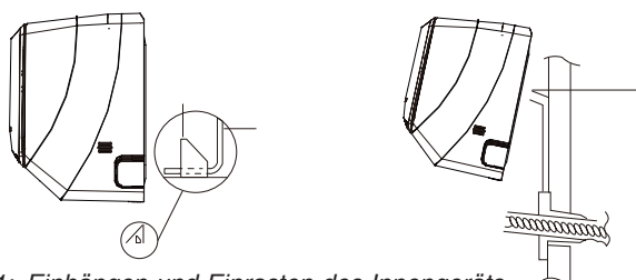
Bild 21: Einhängen und Einrasten des Innengeräts
