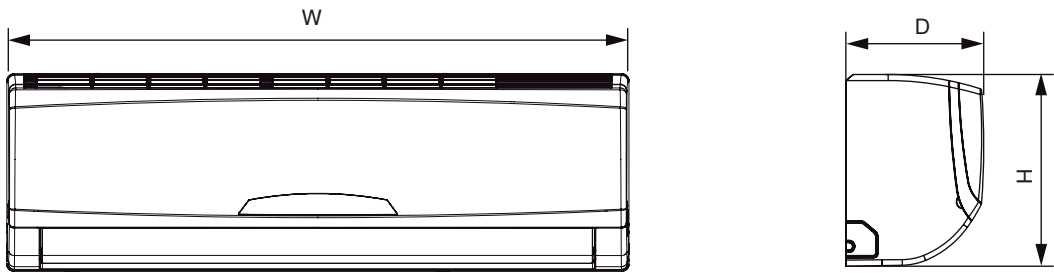
Bild 12: Maßzeichnung Innengeräte Größen 09 - 24
