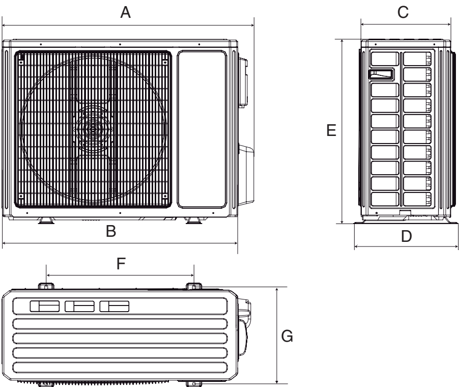
Bild 13: Maßzeichnung der Außengeräte 09 - 24
